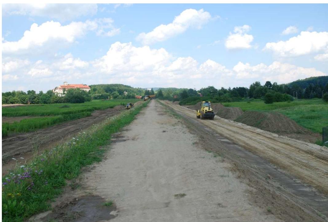
Foto. 21. Zabezpieczenie hałd humusu na Zadaniu 2, stan w trzeciej dekadzie lipca 2020 r. (widok w dół rzeki).
